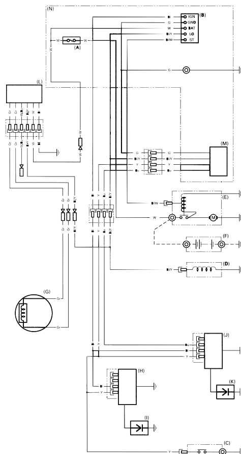
Type à bobine de charge 17 A et avec boîte de commande
