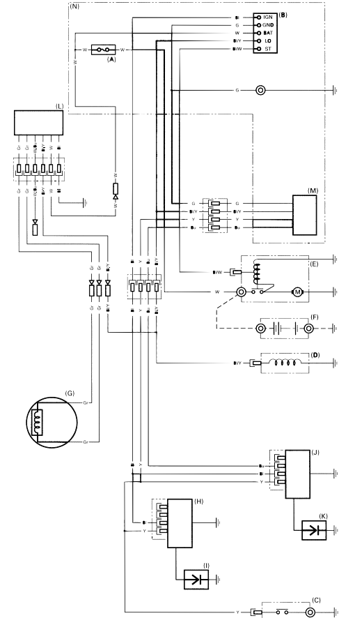
Tipo con bobina de carga de 17 A y con caja de control
